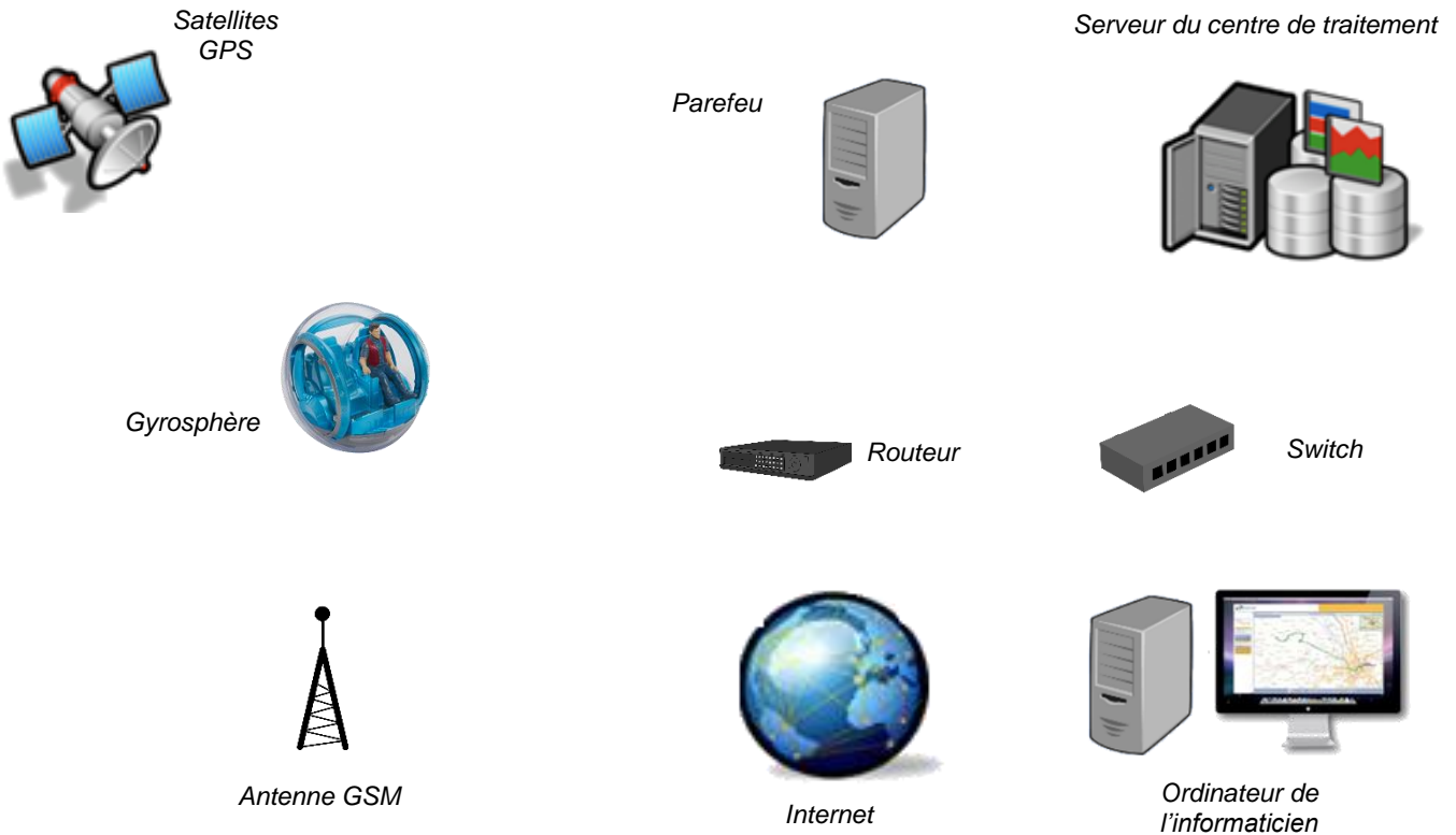
Schéma N°2 – Architecture du système de géolocalisation
